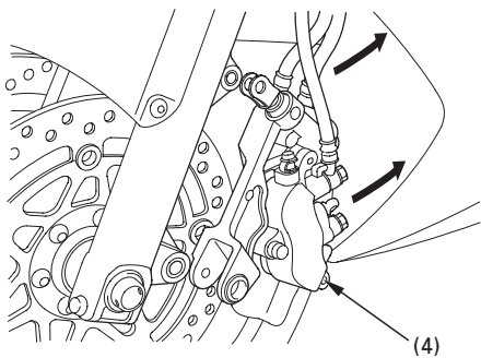
(4) Vasen jarrusylinteri
