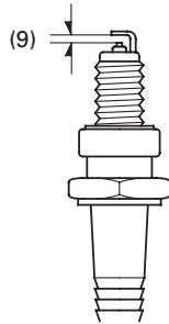
(9) Tulpan kärkiväli
