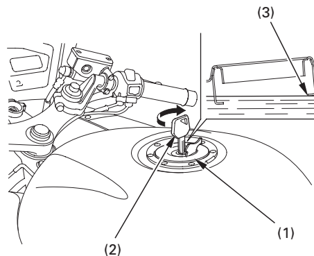
(1) Polttoainetankin korkki (3) Kaula (2) Virta-avain
